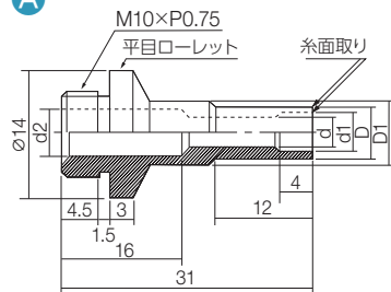
断面図
