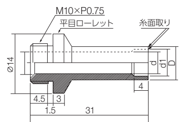
マウスピース断面図B
