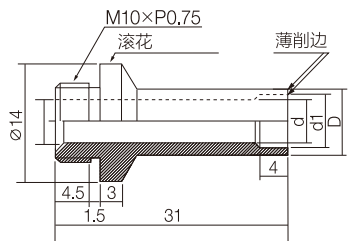
套筒纵向断面图B
