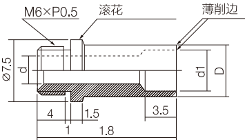
套筒纵向断面图
