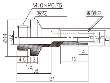
套筒纵向断面图A
